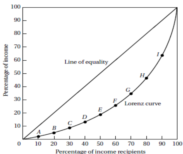
Gambar 1 Kurva Lorenz
